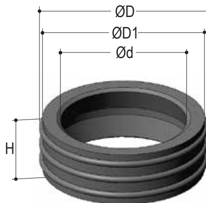
Anel Estanqueador
