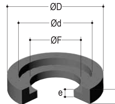
Anel Rebaixado
