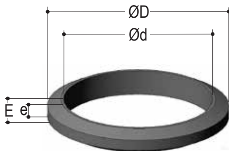
Anel Chanfrado
