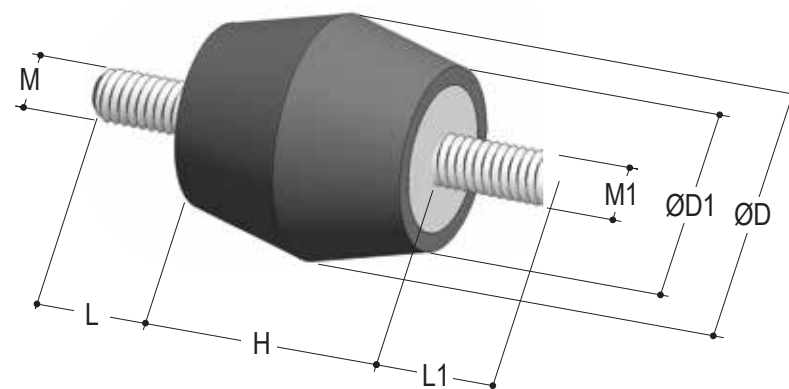
Coxim Bicônico
