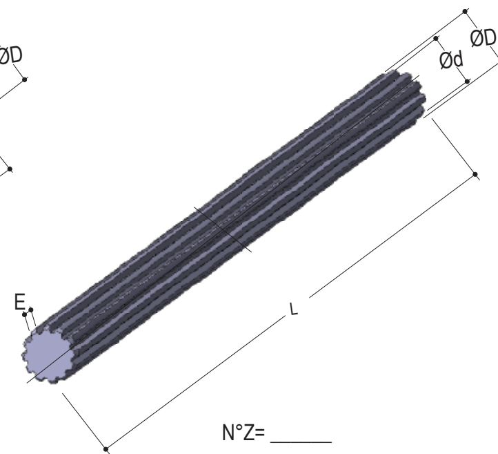
Eixo Ranhurado
