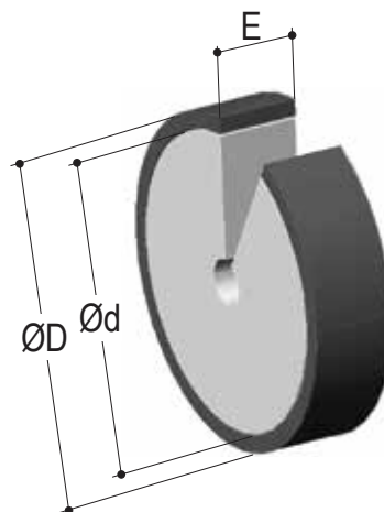
Roldana Plana
