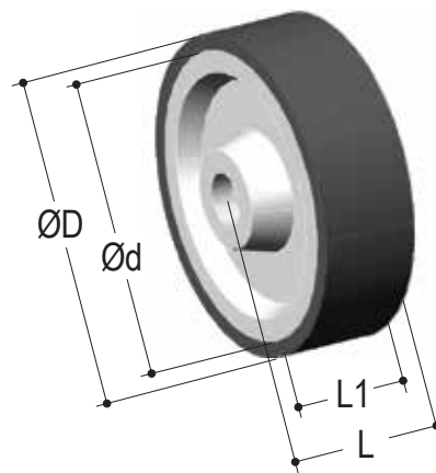
Roda Plana
