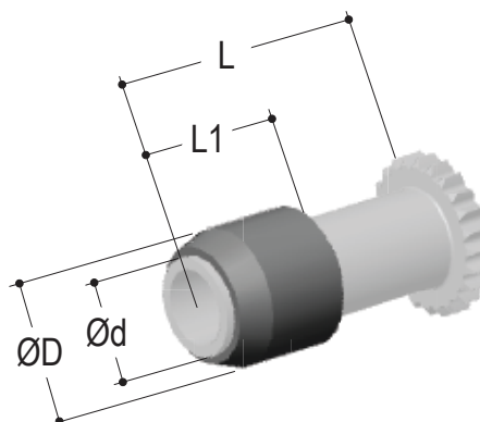
Rolete de Tração
