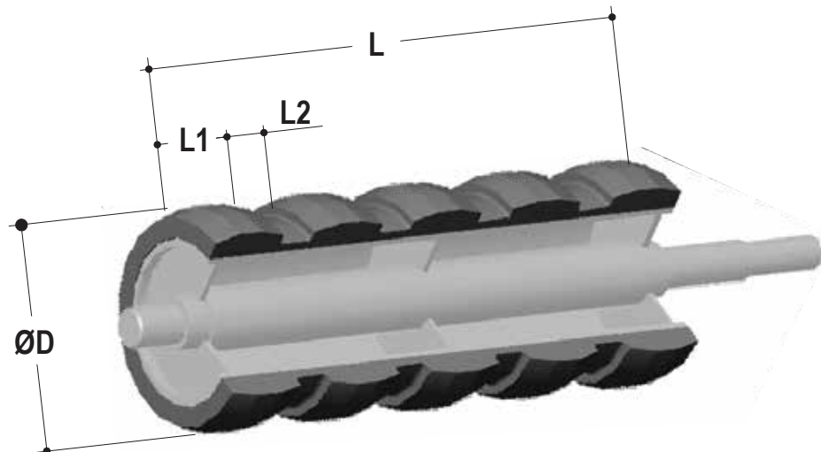
Rolo c/ Canais p/ Correia
