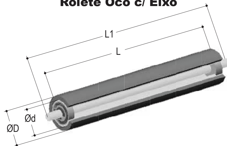
Rolete Oco c/ Eixo
